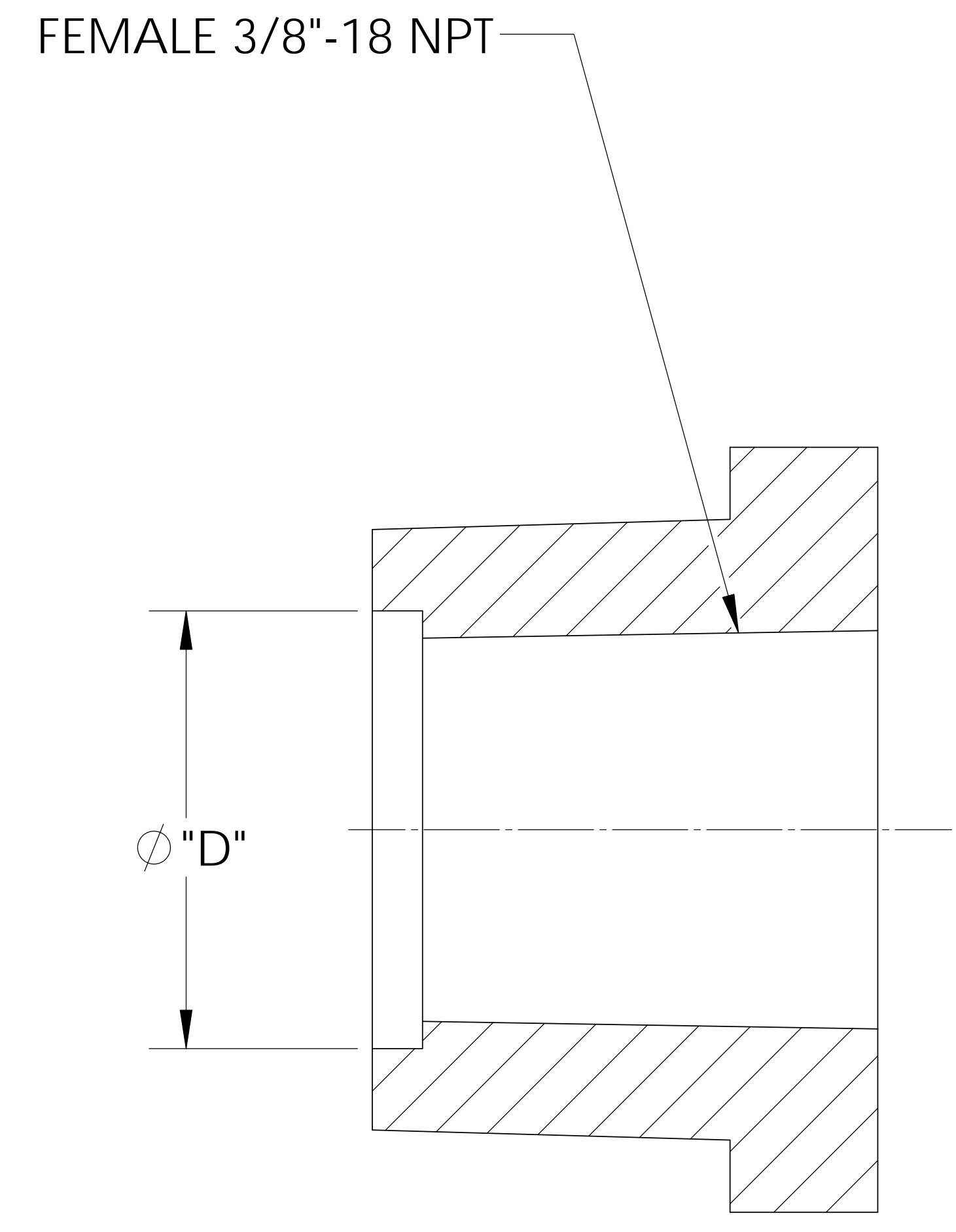
SECTION A-A
